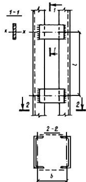
Рис.3. Составной стержень на планках
