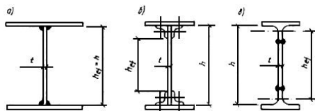
Рис.10. Расчетная высота стенки составной балки
