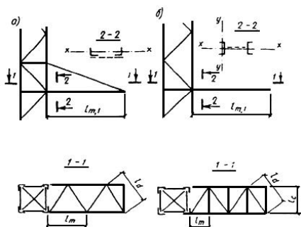
Рис.21. Схемы траверс
